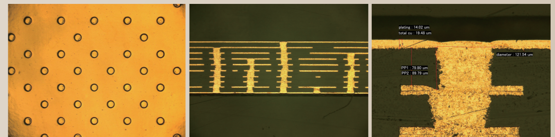
via depth : 80 um / diameter : 120 um / plating : 14.02 um
