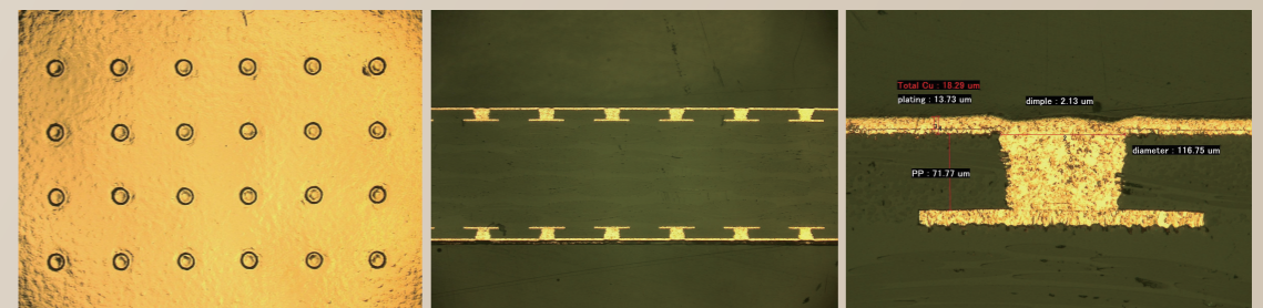
via depth : 70 um / diameter : 120 um / plating : 13.73 um
